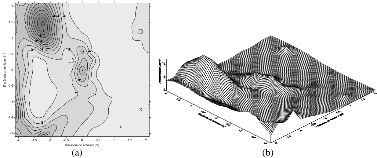
Figura 2. Isoietas (a) e perfil tridimensional (b) do microaspersor Amanco MF 63 L h -1 , operando sob pressão de 200kPa, em condições de campo.
