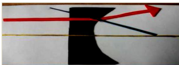
Figura 9- Uma lente de vidro de bordas delgadas, imersa em sulfeto de carbono, é divergente.
