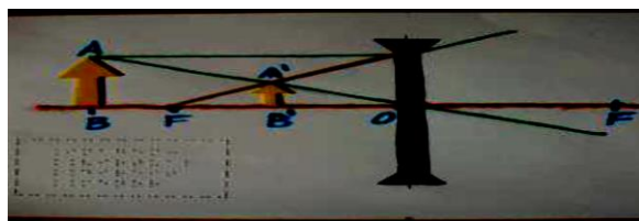
Figura 10 - AB e o objeto real, isto é, objeto luminoso ou iluminado situado diante da lente divergente e A'B' e a imagem projetada.
