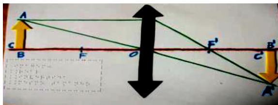
Figura 12 - Objeto real sobre do ponto antiprincipal objeto C
