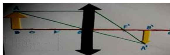
Figura 11 - Objeto real além do ponto antiprincipal objeto C
