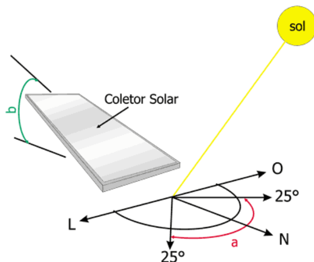
Figura 4 - Posição adequada para o uso do coletor solar (SOUZA, 2000)
