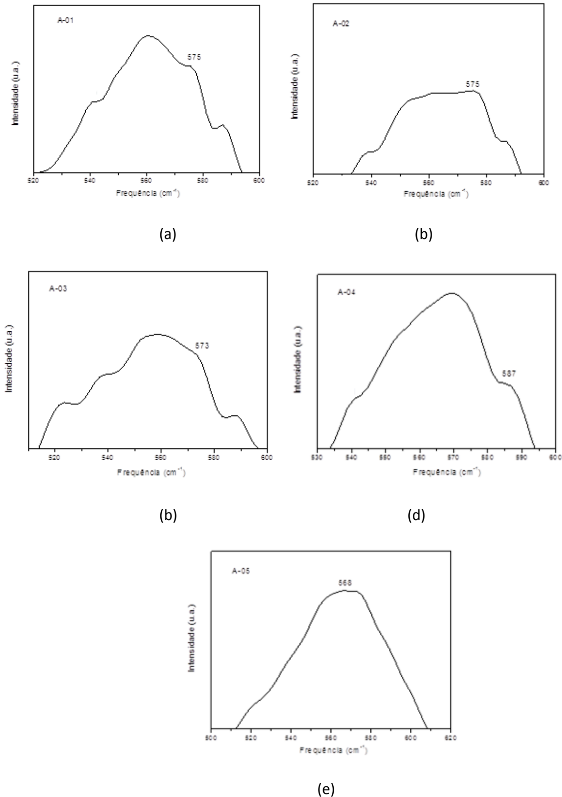
Figura 4: Espectro Raman na região de 500 a 600 \text{cm}^{-1} para as amostras sintetizadas.
