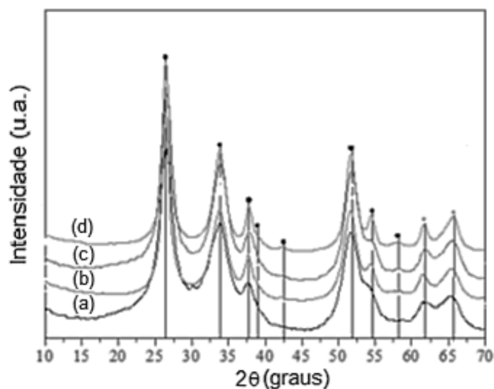
Figura 1: Difratogramas das amostras dopadas com diferentes porcentagens de níquel: (a) A-02, (b) A-03, (c) A-04, (d) A-05 e (•) ICSD-9163-SnO 2 .
