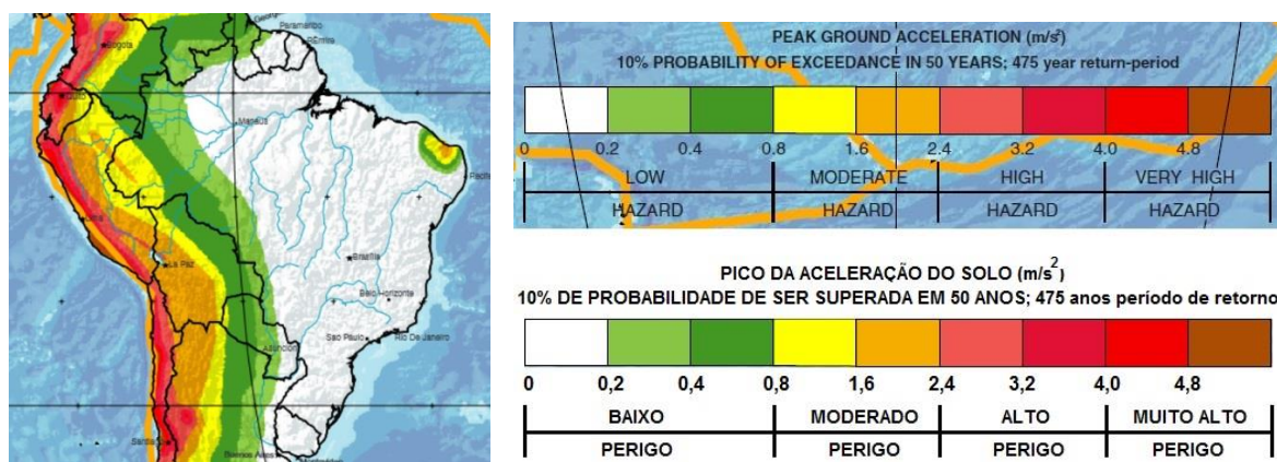
Figura 7: Fração do mapa do perigo sísmico global, destacando-se o Brasil. Fonte: adaptado de GSHAP (1999).
