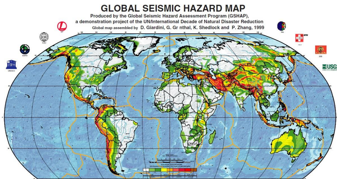
Figura 6: Mapa do perigo sísmico global. Fonte: adaptado de GSHAP (1999).
