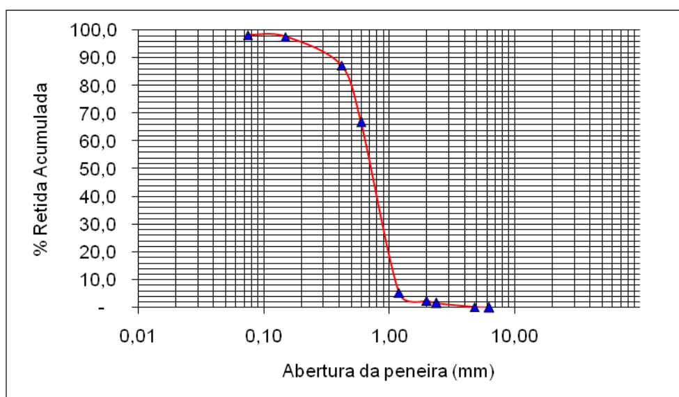
Figura 3 – Curva granulométrica do arisco.
