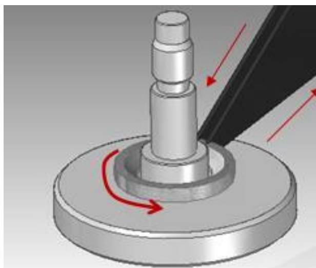
Figura 3. Dispositivo utilizado no processo de têmpera tipo: Indutor Reto com Furo \varnothing 34mm (Mod. Fab. KRM "R" - Base: \varnothing 30,3 Haste), indicando o virabrequim sendo processado termicamente. (Fonte: Fabricante da motocicleta).
