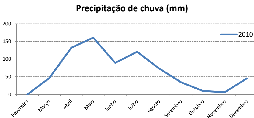
Figura 5 - Gráfico mostrando a precipitação de chuva em 2010 FONTE: [17].
