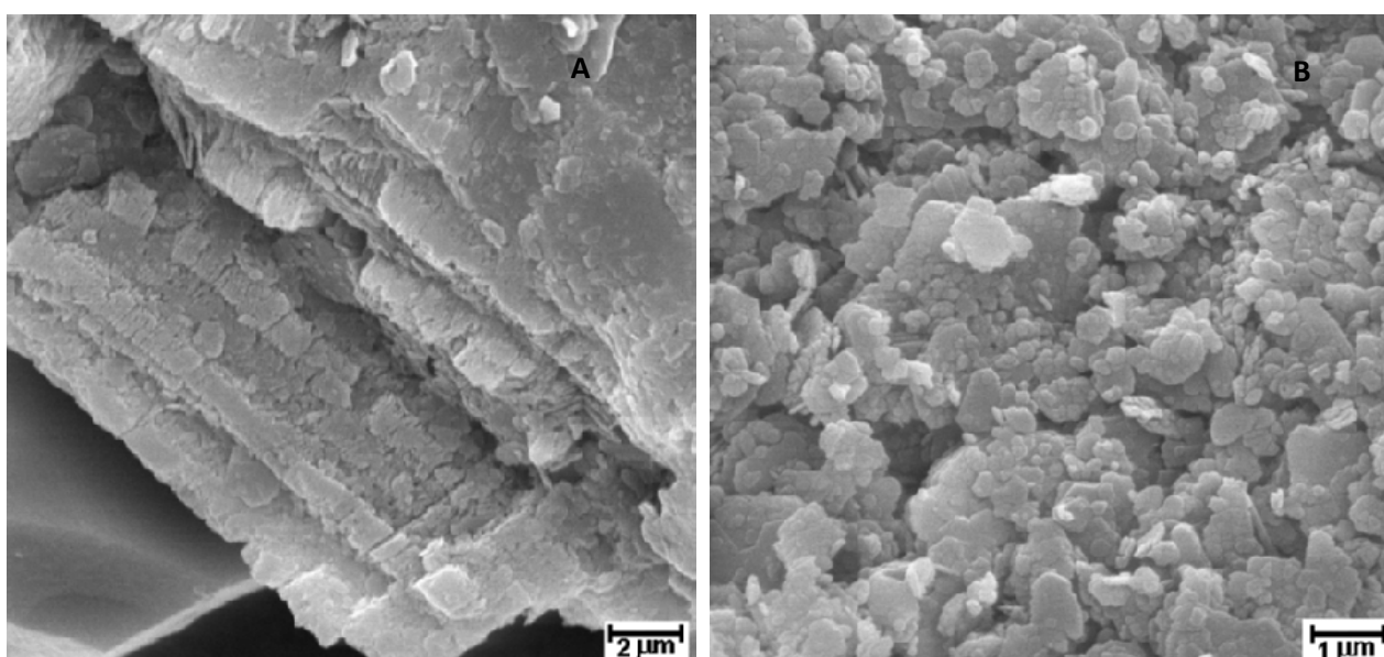
Figura 3. Imagens do caulim MPC01. A- antes do beneficiamento; B- após o beneficiamento.
