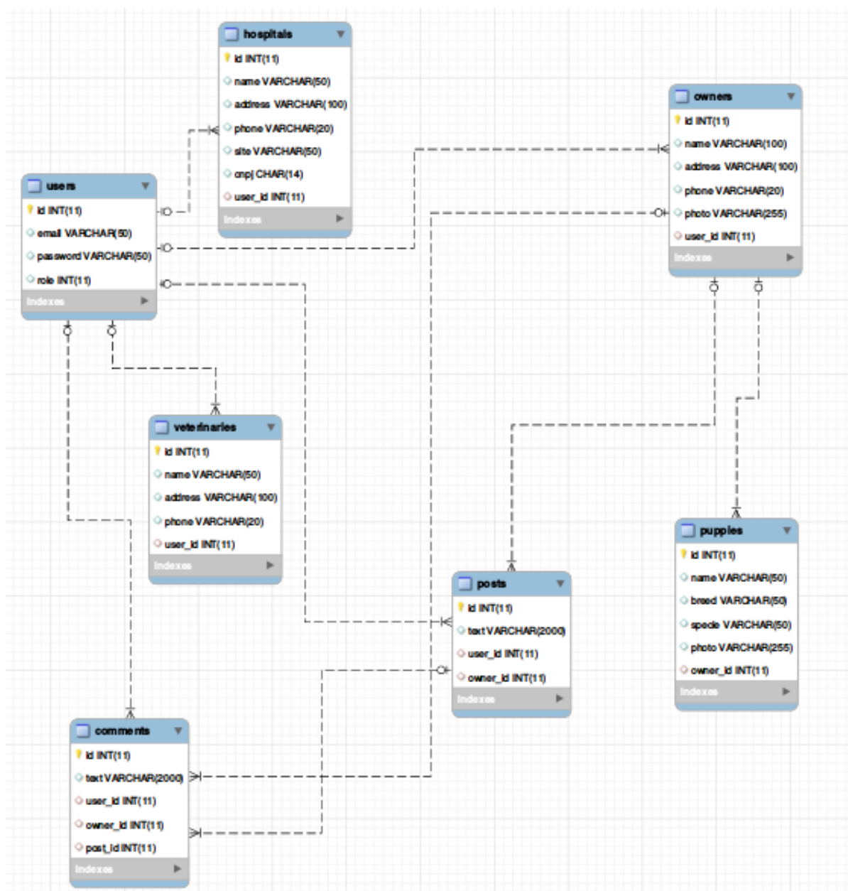
Figura 5: Diagrama Entidade-Relacionamento
